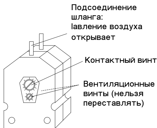
Выключатель давления
